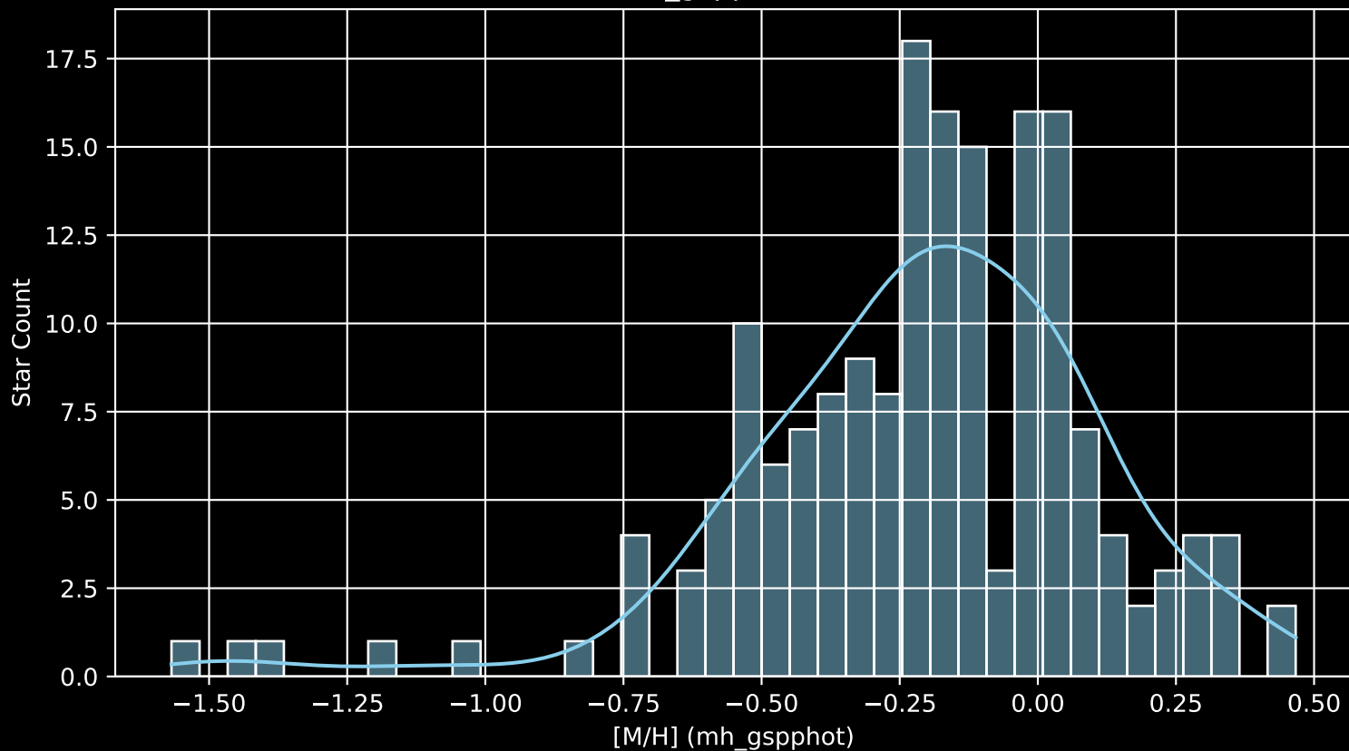
APOGEE DR17 Field: [048+88 MGA [M/H] (mh_gspphot) (n= 176)
